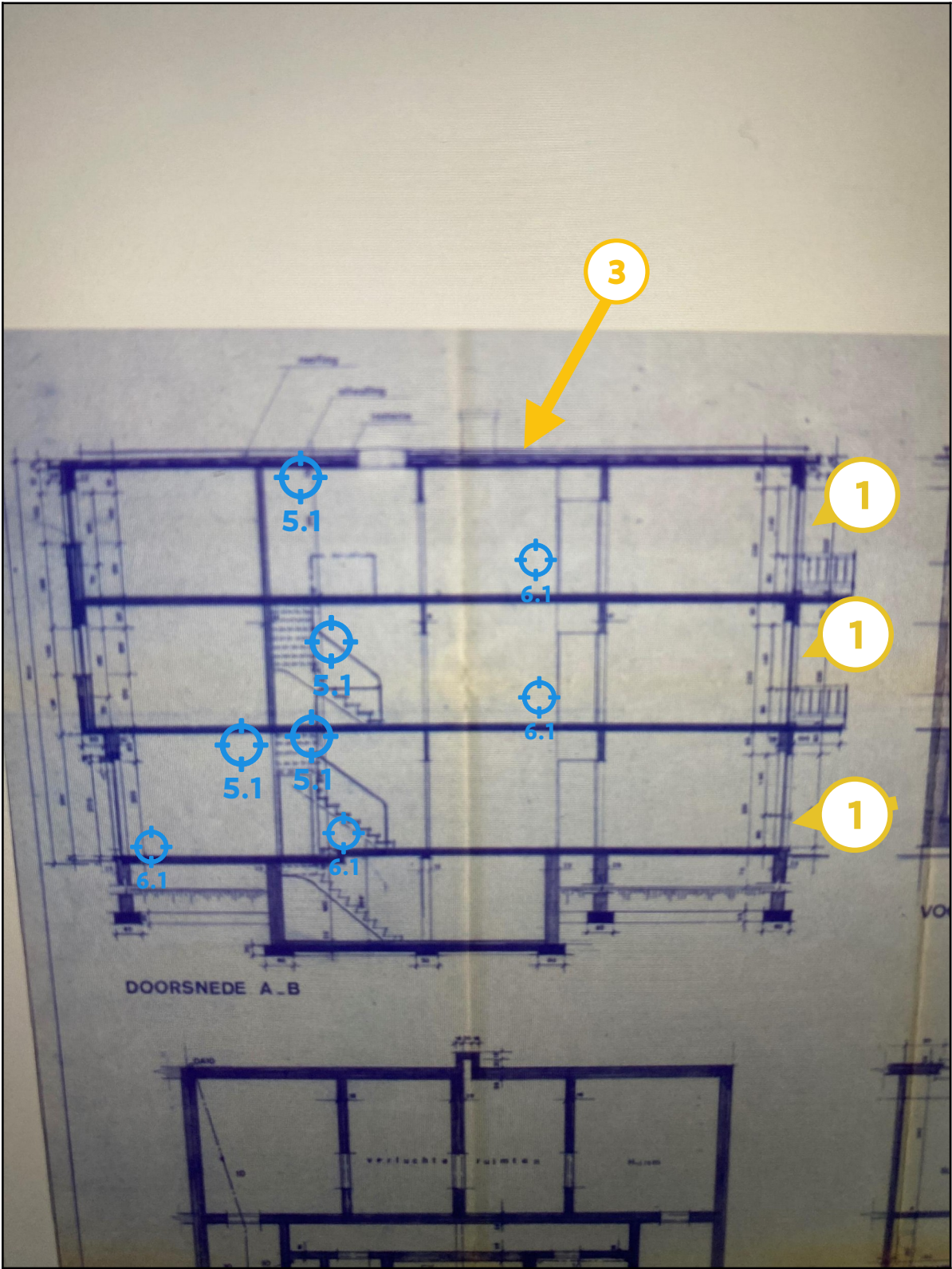
Legende van plan 1.3: Doorsnede Plan
